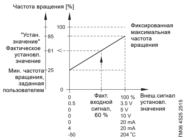
Рис. 76 Пример влияния установленного значения с постоянной характеристикой
