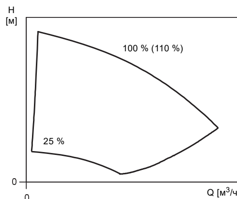
Рис. 20 Рабочий диапазон насосов TPE Серия 2000
