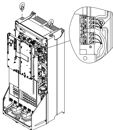
Рис. 170 Клеммы для подключения реле, C1
