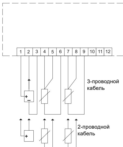
Рис. 171 Схема электрических соединений, MCB 114
