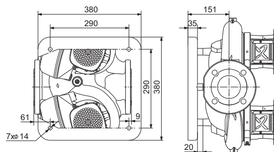
Чертеж, TPE2 D, TPE3 D 100
