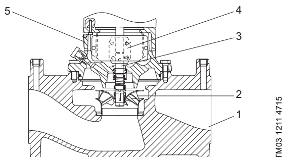
Рис. 12 Чертеж насоса TP Серия 200 (с фланцевым соединением) в разрезе
