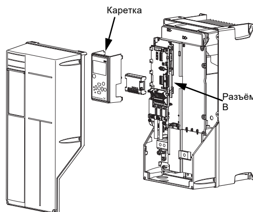
Рис. 172 Корпусы B2, C1
