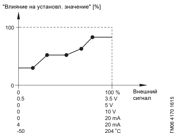
Рис. 79 "Таблица влияния", пример с пятью точками
