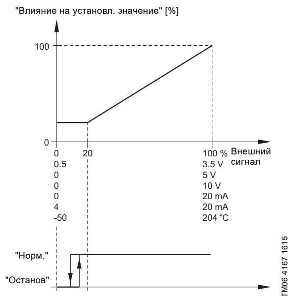
Рис. 78 "Линейная функция с остановом"
