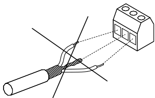
Рис. 154 Не скручивайте экран
