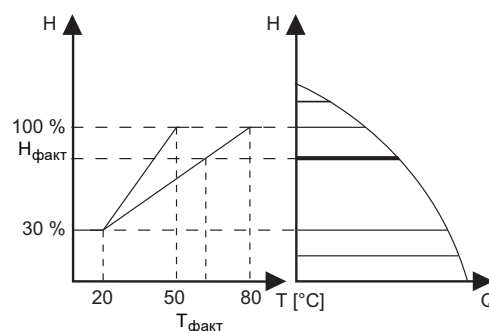
Рис. 81 "Влияние температуры"
