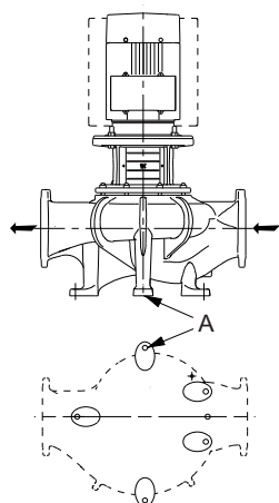
Рис. 173 Принципиальная схема насоса Серии 300, предназначенного для монтажа на опорах (А)
