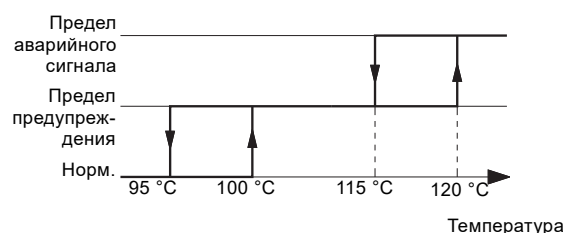
Рис. 124 Контроль температуры подшипников с использованием предельных значений для предупреждений и аварийных сигналов
