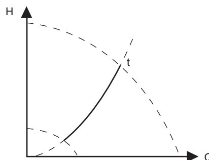
Рис. 56 "Постоянная температура"
