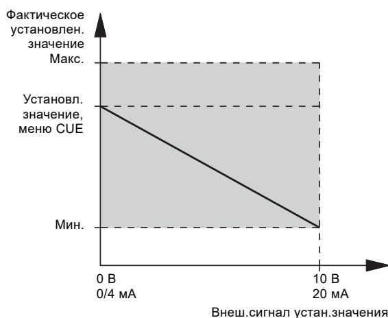
Рис. 108 Обратный внешний сигнал установленного значения
