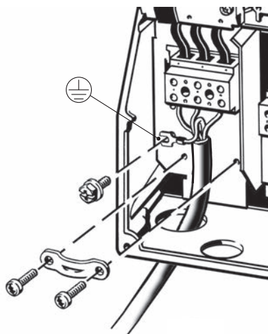
Рис. 158 Подключение питания, В2
