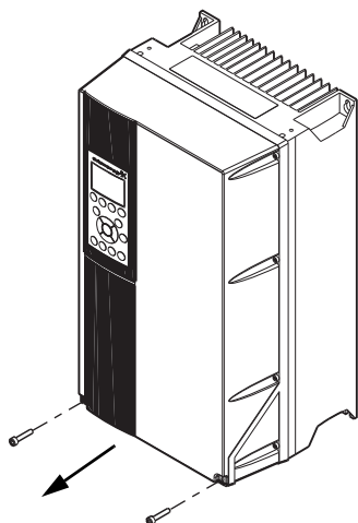
Рис. 163 Доступ к сигнальным клеммам, В2 и С1
