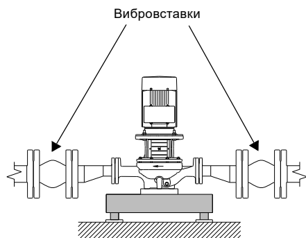
Рис. 140 Насос TP с вибровставками большого размера
