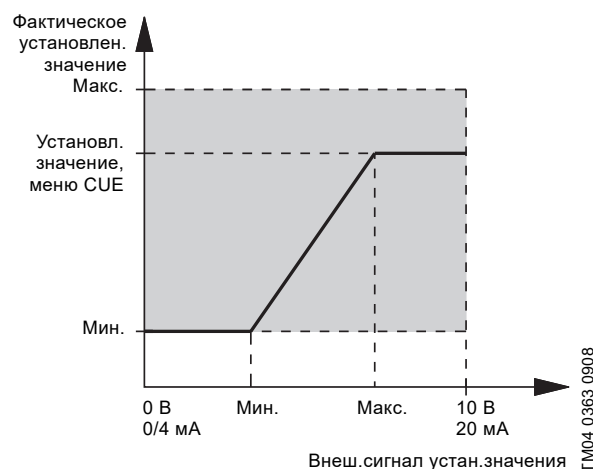
Рис. 107 Сокращенный внешний сигнал установленного значения
