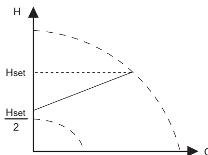
Рис. 52 "Пропорциональное давление"
