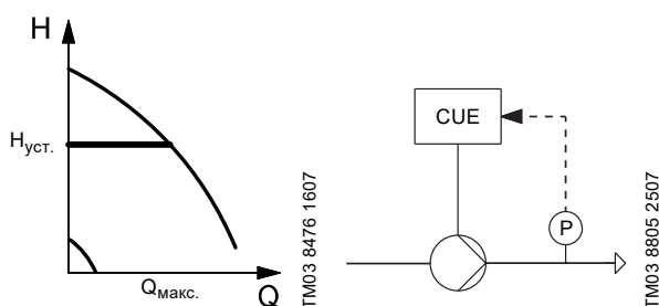
Рис. 89 Постоянное давление
