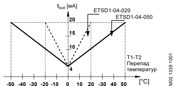
Рис. 177 Характеристики датчика
