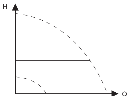
Рис. 54 "Постоянное давление"
