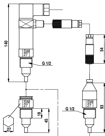
Рис. 178 Габаритный чертеж
