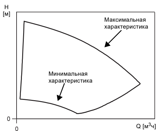
Рис. 127 Минимальная и максимальная кривые характеристики
