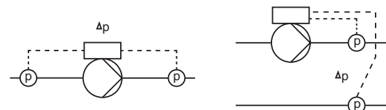
Рис. 59 "Постоянный перепад давления"
