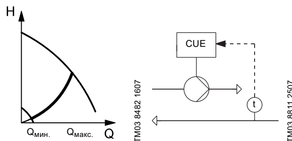
Рис. 104 Постоянная температура
