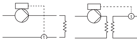
Рис. 57 "Постоянная температура"
