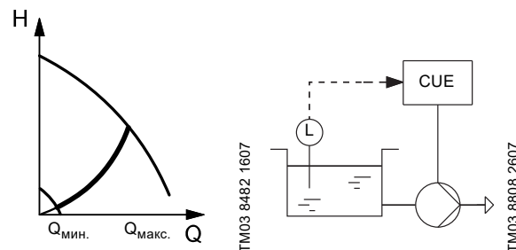
Рис. 101 Постоянный уровень
