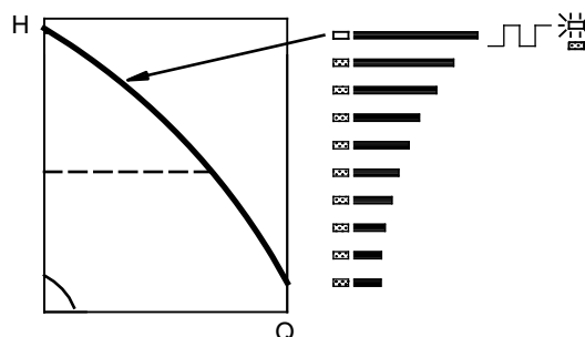
Рис. 37 Максимальная характеристика
