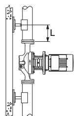
Рис. 133 Монтаж насоса на трубопроводе
