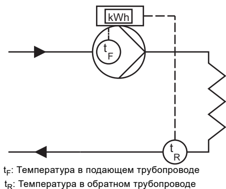
Рис. 48 Пример: Насос установлен в подающем трубопроводе, дополнительный датчик температуры установлен в обратном трубопроводе
