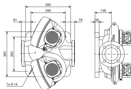
Чертеж, TPE2 D, TPE3 D 100
