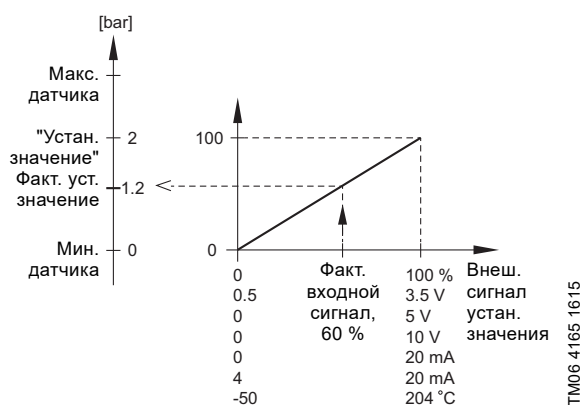
Рис. 75 Пример изменения установленного значения по сигналам с датчиков
