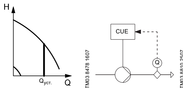
Рис. 100 Постоянный расход
