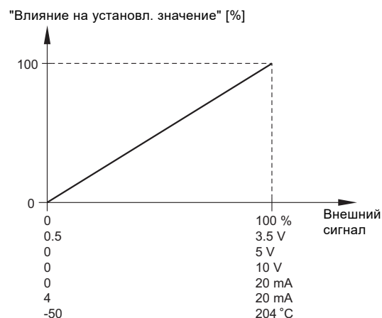
Рис. 77 "Линейная функция"
