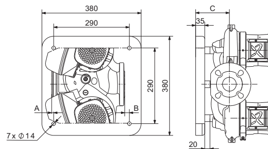
Чертеж, TPE2 D, TPE3 D 80
