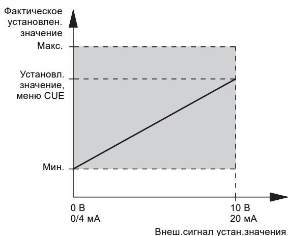
Рис. 106 Внешнее установленное значение
