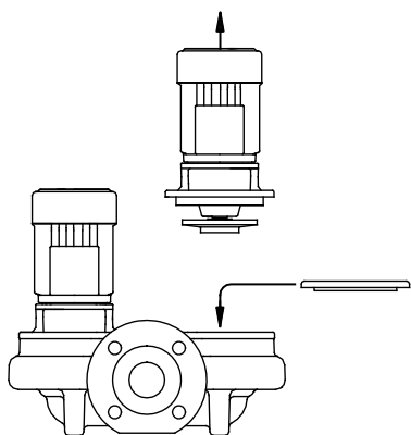
Рис. 174 Глухой фланец
